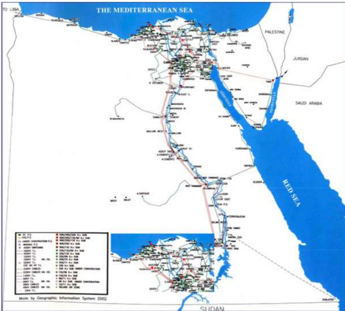
Fig. 1.The Egyptian grid [20].
