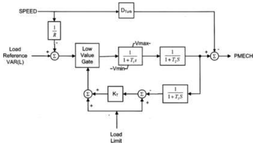
Fig. 3.GASTmodel.
