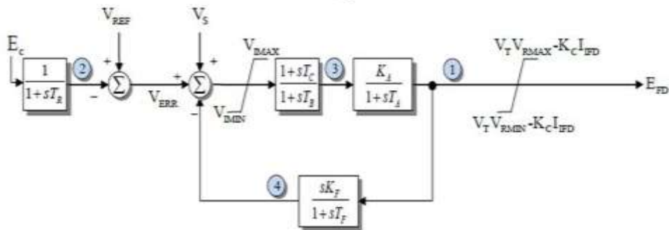
Fig. 5.EXST1model.
