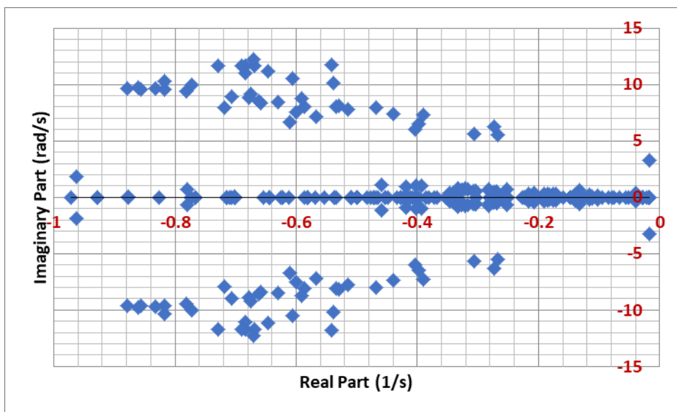
Fig. 6. Critical eigenvalues.
